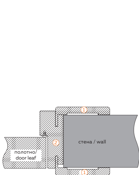
Схема монтажа без использования добора Adjustable door frame
